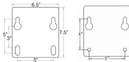
Mounting Plate (GBA-180)
