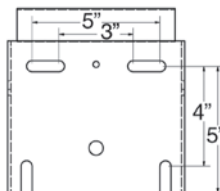
Mounting Plate (GBA-648, GBA-548)
